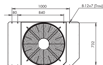
Vista superiore
