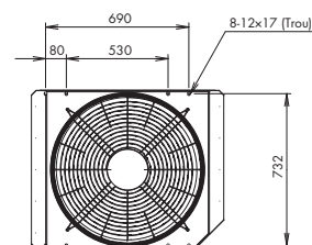
Vista superiore
