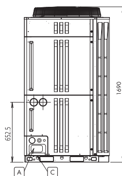
Vista frontale
